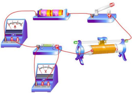
图2-4 欧姆定律实验简化示意图
