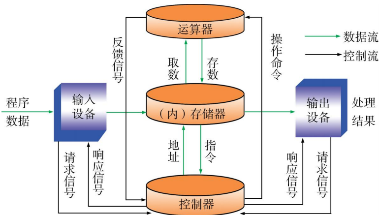
图3-10 计算机程序运行图
