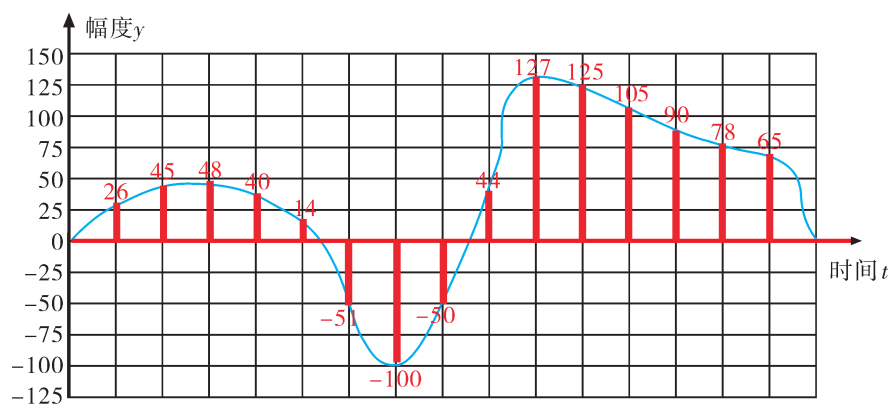
图1-12 脉冲幅度调制信号的量化
