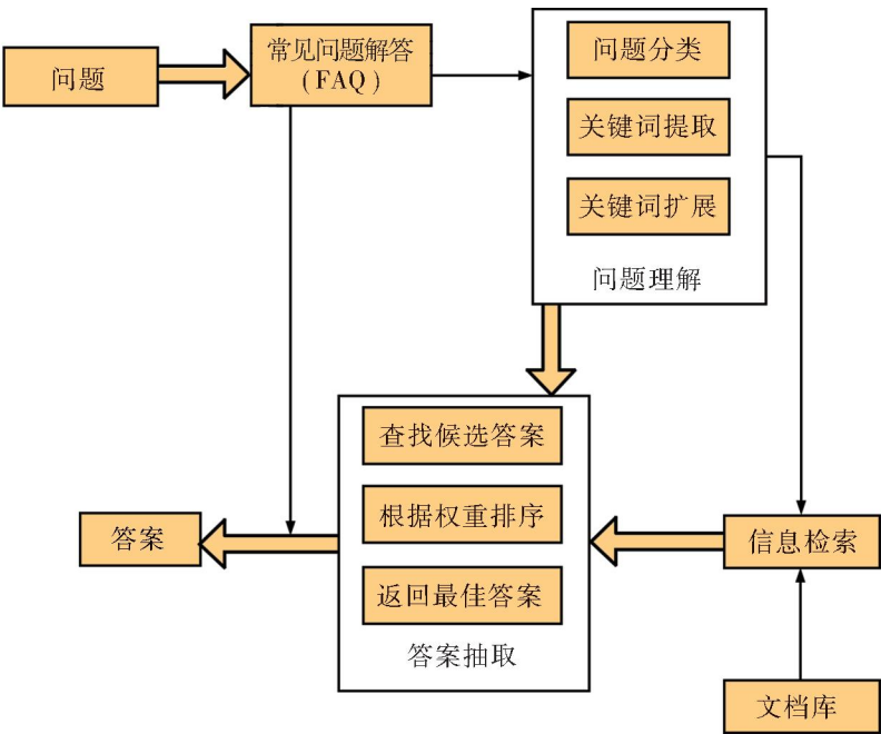
图6-5 典型的智能问答系统结构示意图
