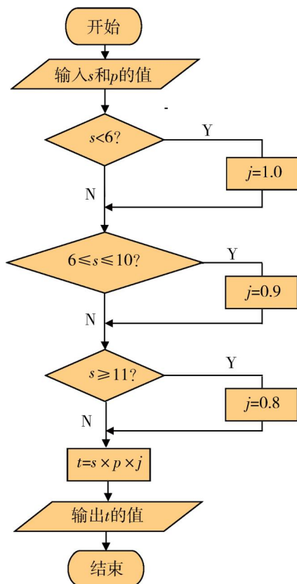
图4-8 网购笔记本的金额计算流程图
