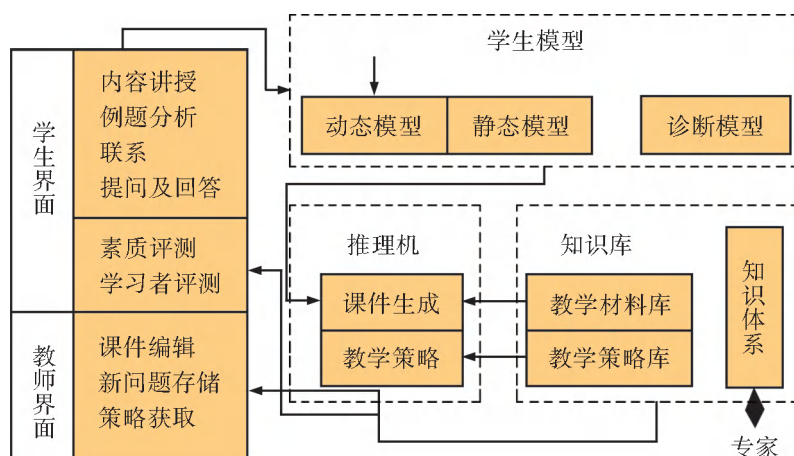
图6-11 智能导师系统结构模型
