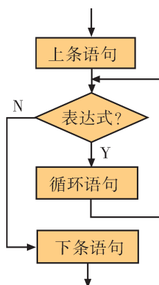
图4-15 while循环执行过程流程图
