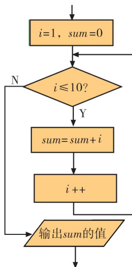
图4-14 累加算法流程图
