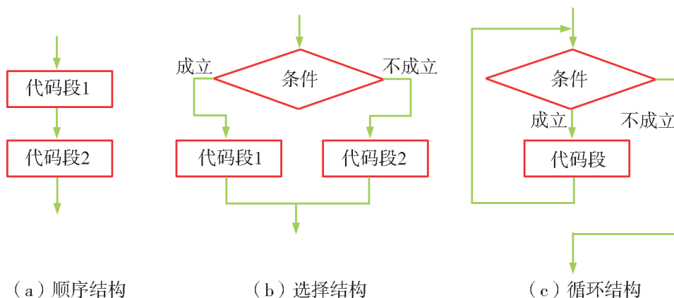
图3-9 三种基本控制结构
