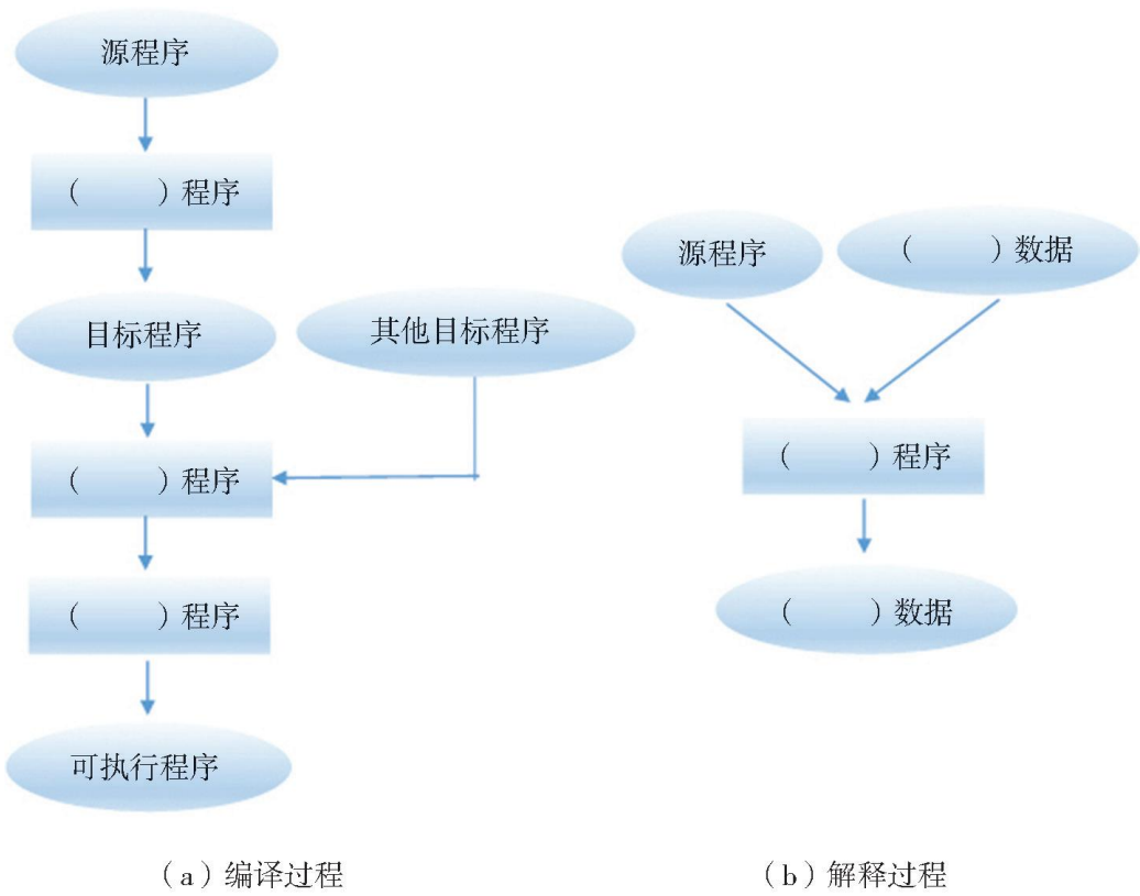
图3-15 编译过程和解释过程
