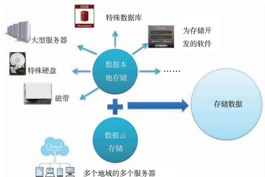
图5-6 数据的存储
