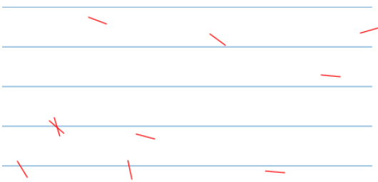
图2-10 投针实验
