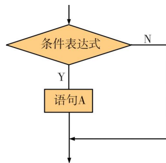
图4-7 if语句的执行过程
