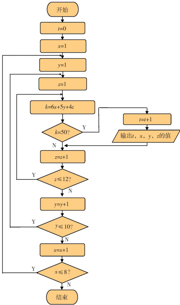
图3-8 求方程正整数解的流程图
