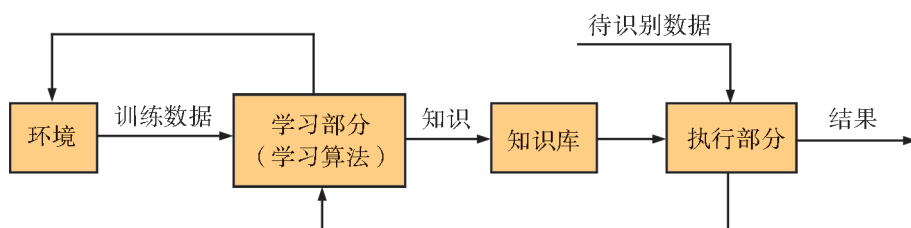
图6-9 训练模型程序的逻辑结构
