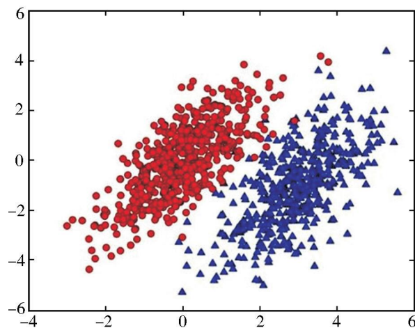
图5-11 数据分布
