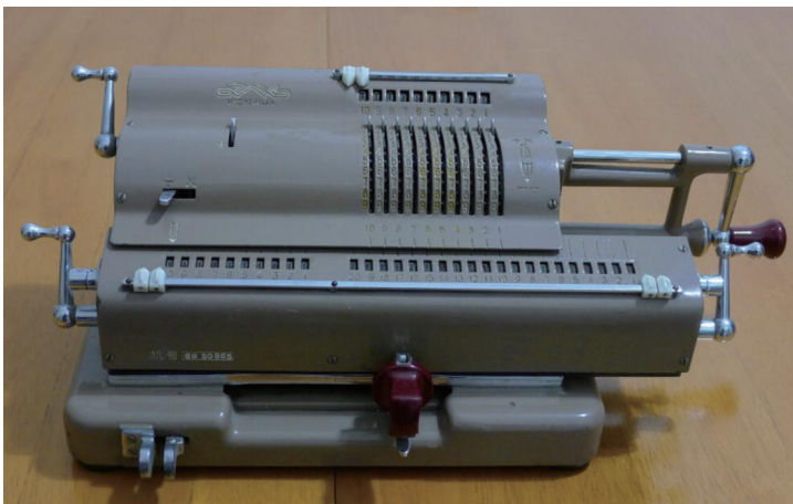
图3-16 手摇计算器
