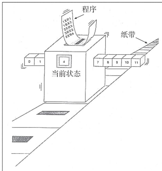
图1-14 图灵机模型
